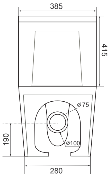
Vista trasera
